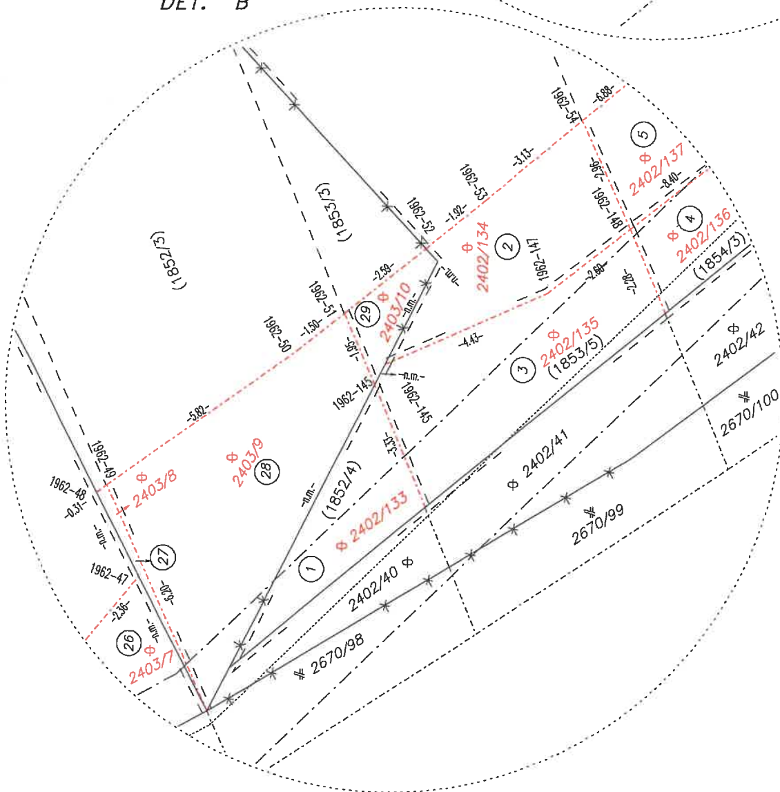
DET. "B"
